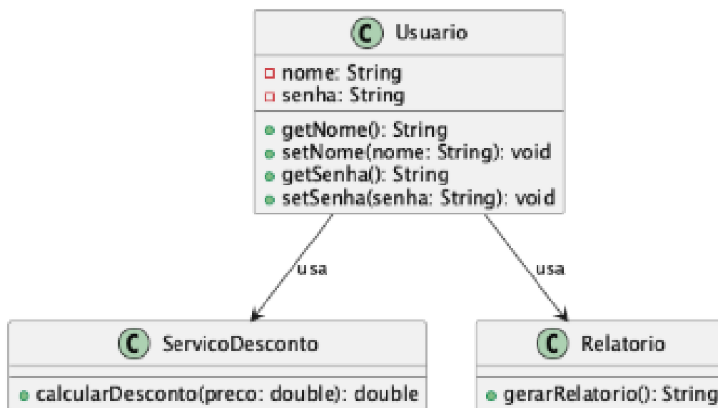
Figura 3 – diagrama de classes
